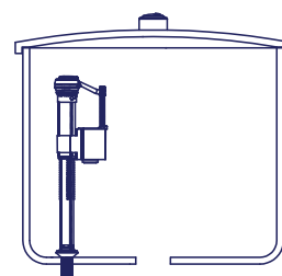
INSTALACIÓN VÁLVULA
